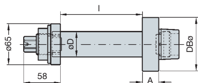
Оправка для фрез HSK 85 WS с гайкой шпиндельной
