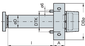
Оправка для фрез HSK 85 WS с зажимным винтом
