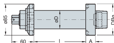
Оправка для фрез HSK 85 для гидравлической втулки с гайкой шпиндельной
