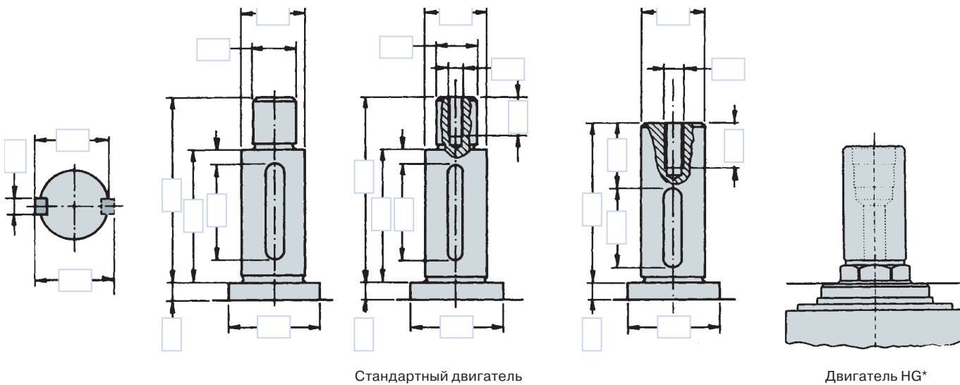
Стандартный двигатель
