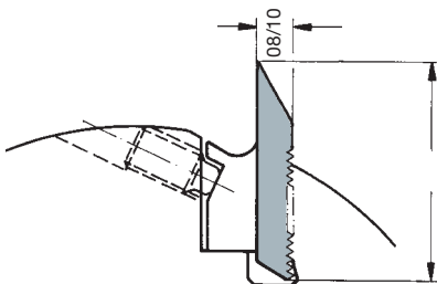
Фреза сборная профильная толщина ножа 8 – 10 мм
