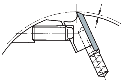
Фреза сборная с системой прижимных клиньев
