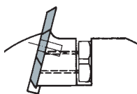
Клин прижимной с винтом для радиусных ножей HS
