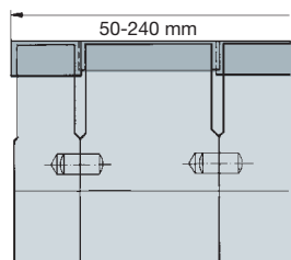
Фреза сборная для обработки плоских поверхностей, модульная система
