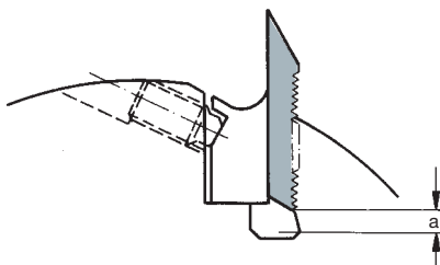
Фреза сборная профильная толщина ножа 6 мм
