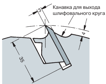
Фреза сборная для обработки плоских поверхностей Hydro RotaPlan Высота ножа 35 мм
