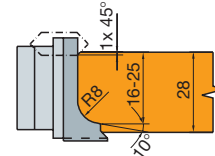
Образец профиля P3
