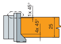
Образец профиля P4
