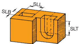
Направляющая шина
