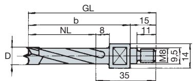
Сверло спиральное, хвостовая часть с резьбой
