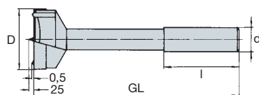
Сверло с цилиндрической головкой
