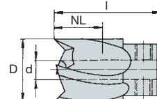
Зенкер 180°
