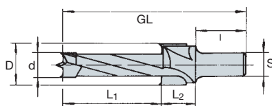
Сверло ступенчатое
